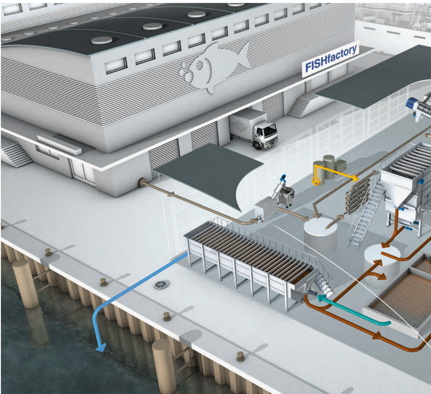
Maschinen und Einsatzgebiete der HUBER-Maschinenteknik im Abwasserprozess der Fischindustrie
