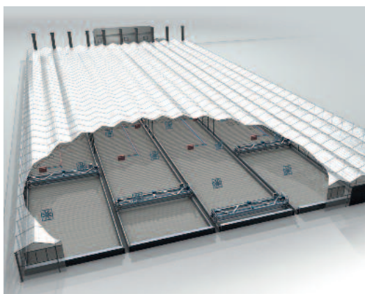
Gesamtansicht solare Trocknung
