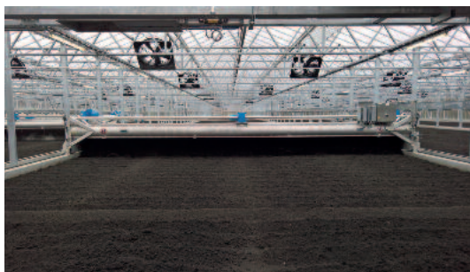
HUBER Schlammwender SOLSTICE® im Wendebetrieb
