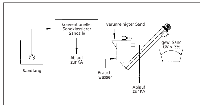
Verfahrensschema
