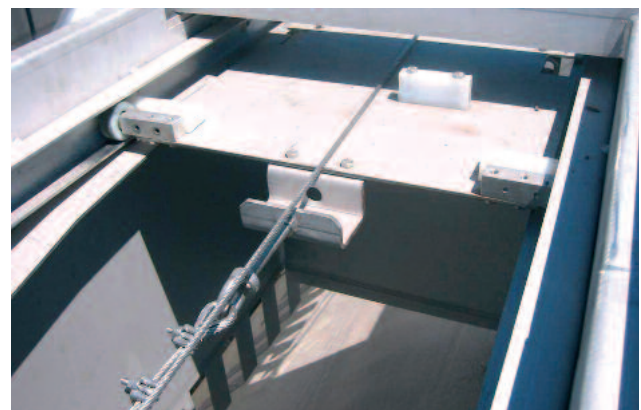
Automatische Fetträumung mittels Fettpaddel
