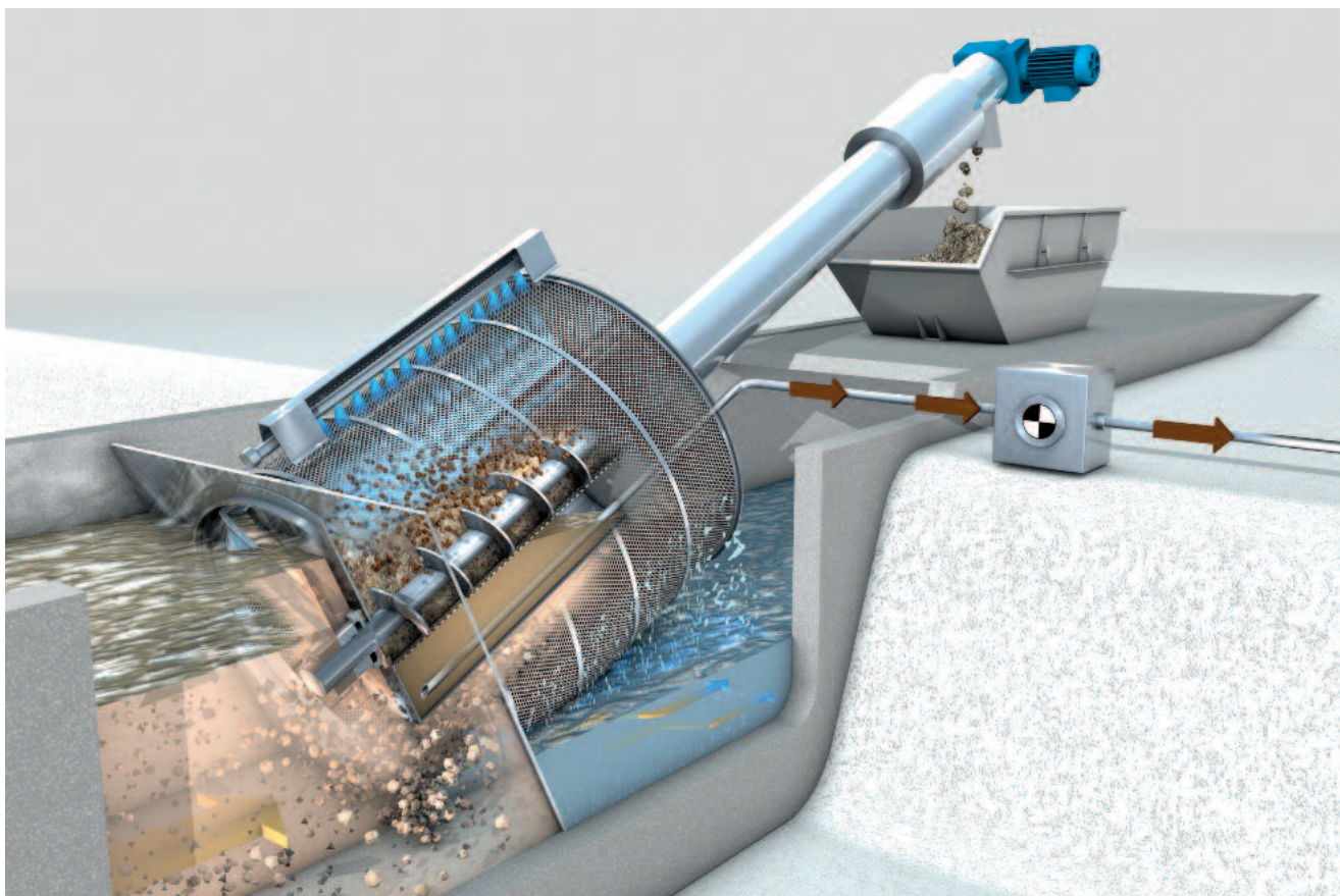
Prinzipdarstellung des Feinstsieves ROTAMAT® Membrane Screen RoMem
