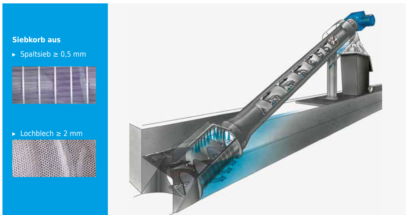
Schematische Darstellung der HUBER Siebschnecke ROTAMAT® Ro9.
