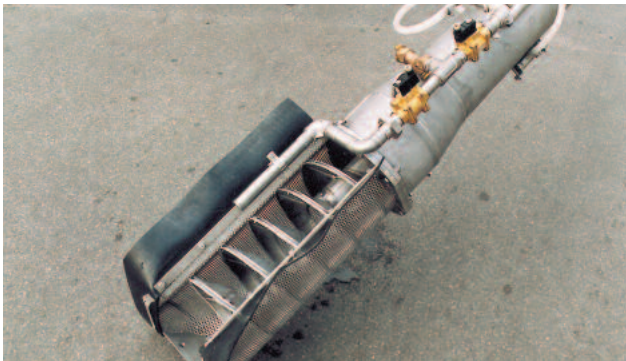
Integrierte Rechengutauswaschung (IRGA). Durch das ROTAMAT®-Prinzip ist es möglich, die Rechengutauswaschung direkt in den unteren Steigrohrbereich zu integrieren.
