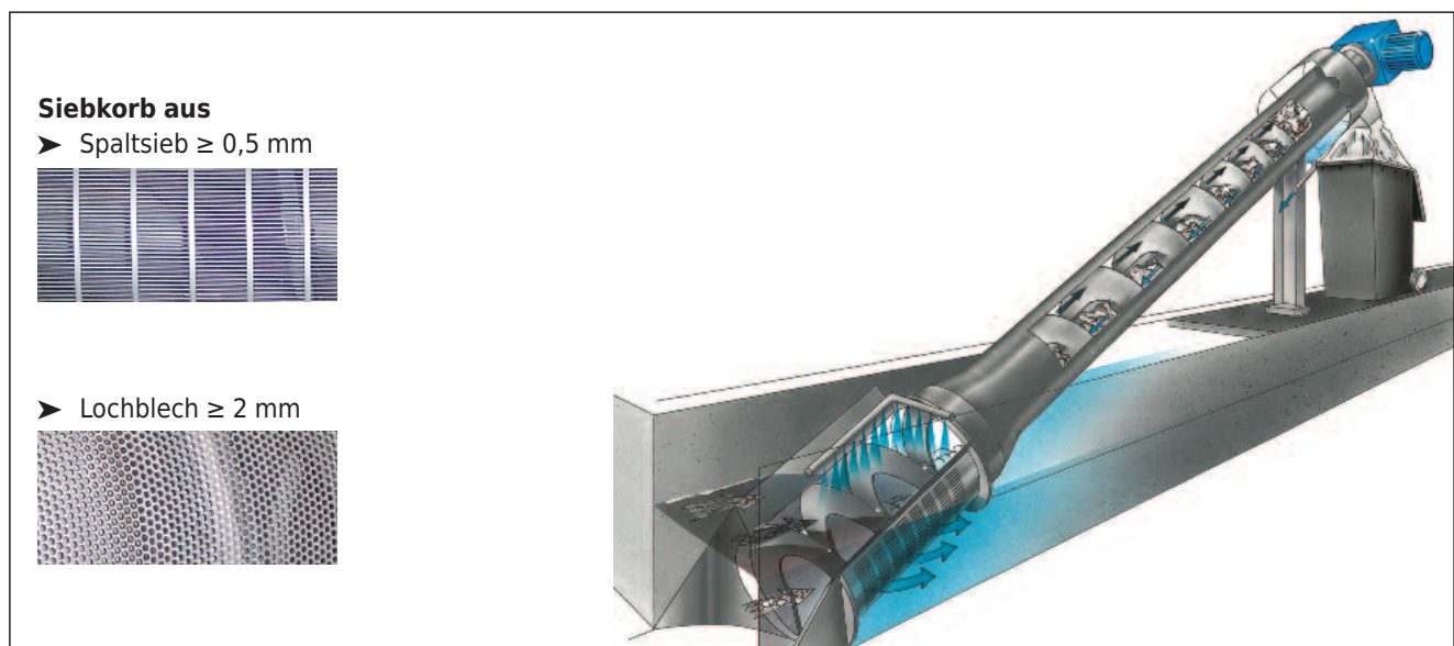
Schematische Darstellung der HUBER Siebschnecke ROTAMAT® Ro9
