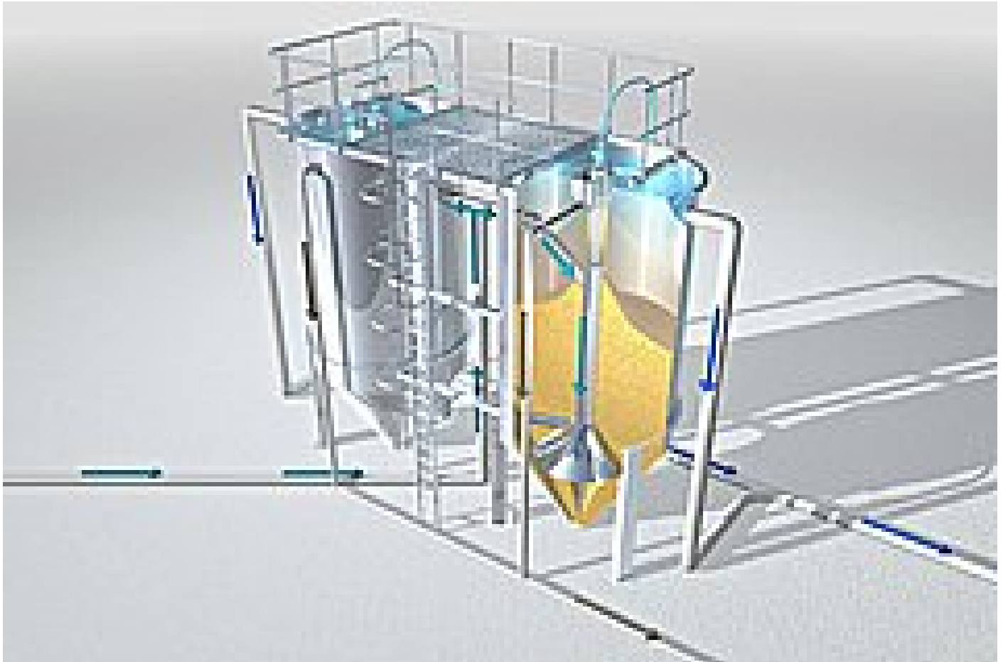
Funktionsprinzip des HUBER Sandfilters CONTIFLOW®
