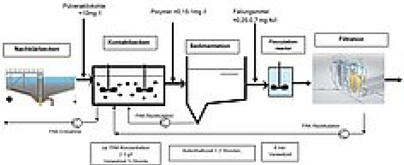
Gängige Verfahrenstechnik der vierten Reinigungsstufe mit Pulveraktivkohle
