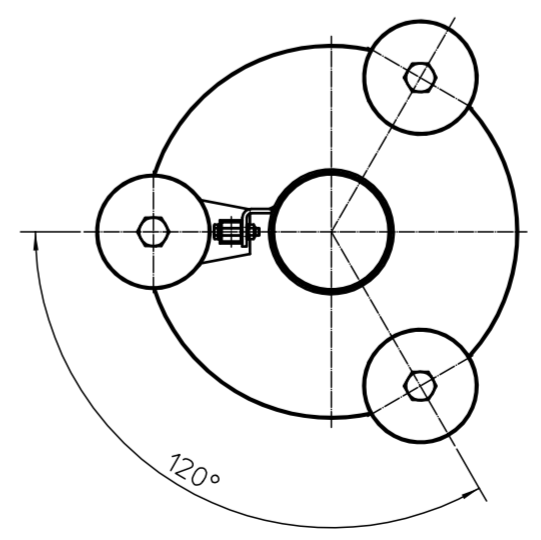
Schnitt/section: A-A
