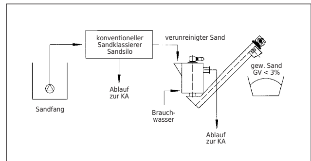
Verfahrensschema
