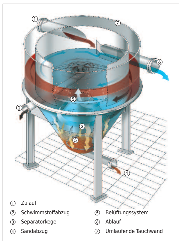
Prinzipskizze des HUBER Rundsandfanges HRSF
