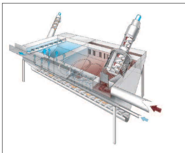
Prinzipskizze der ROTAMAT® Kompaktanlage Ro 5HD
