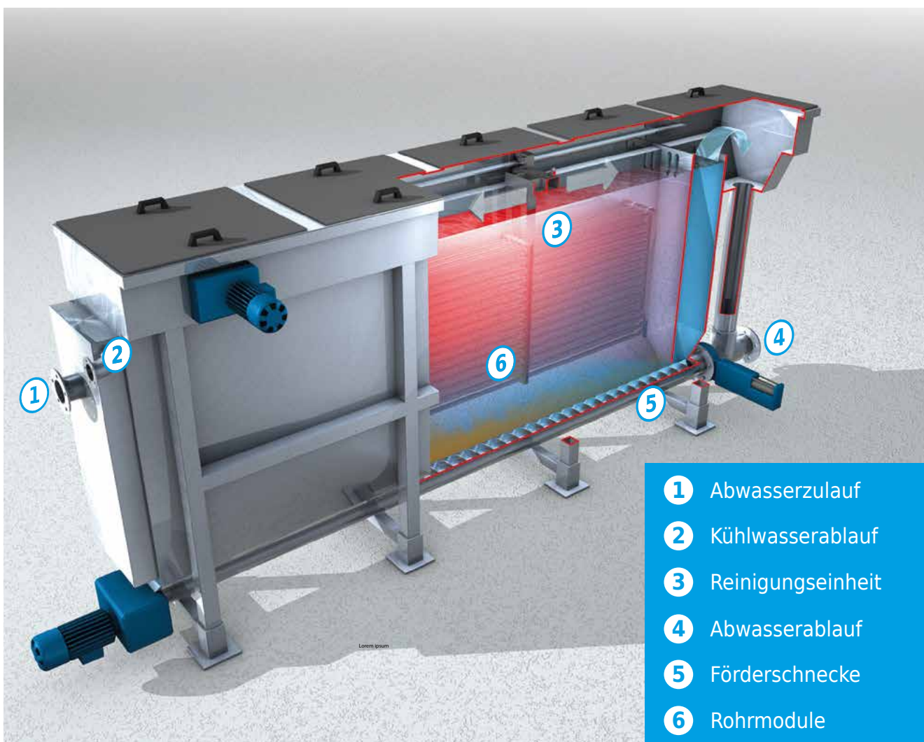
Schematische Darstellung des HUBER Abwasserwärmetauschers RoWin.
