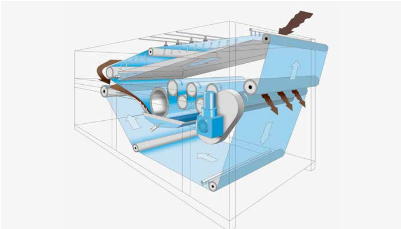
HUBER Bogenpresse B-PRESS mit 8 Walzen-Presszone.
